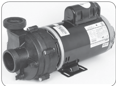
Pompa con Motore (può variare per modello)
