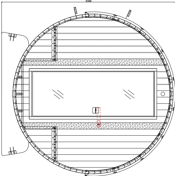
前外主视图
