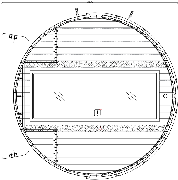
前外主视图
