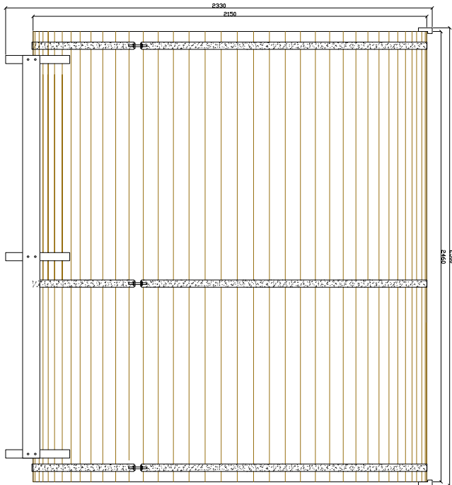
侧视图
