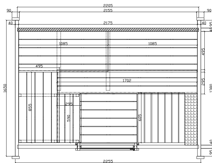
前外观视图
