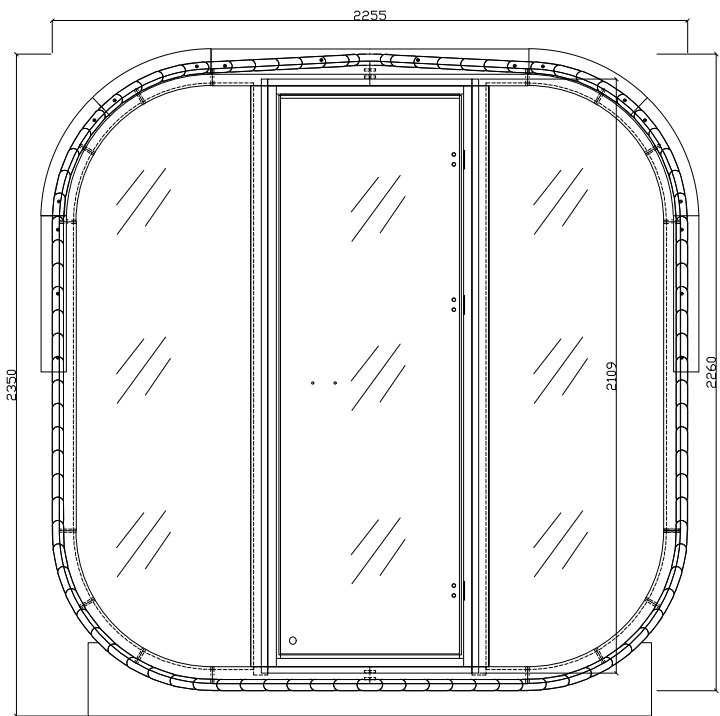
前外观视图
