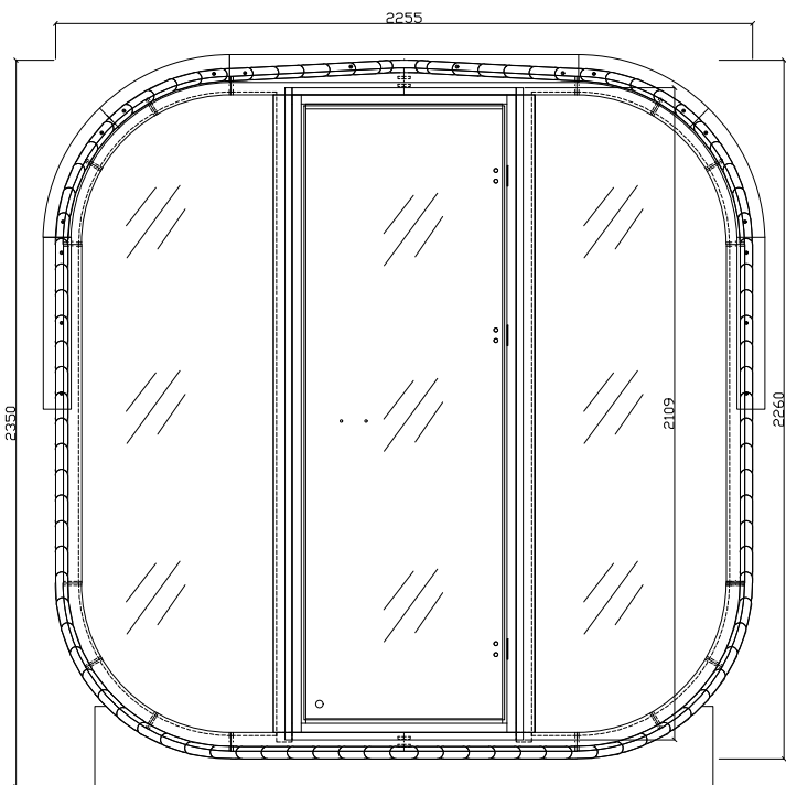
前外观视图
