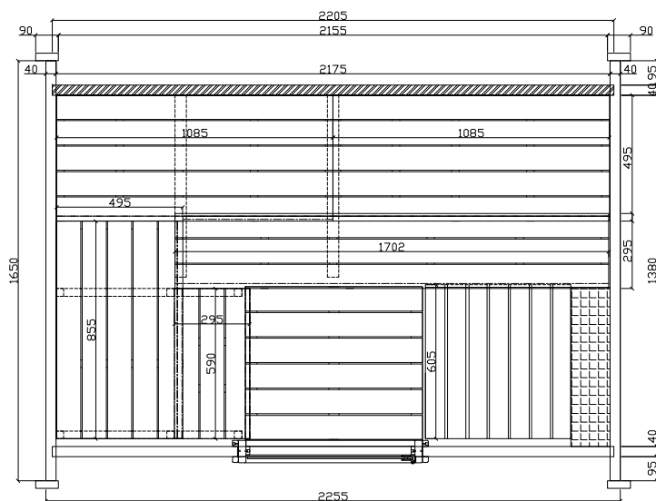
前外观视图
