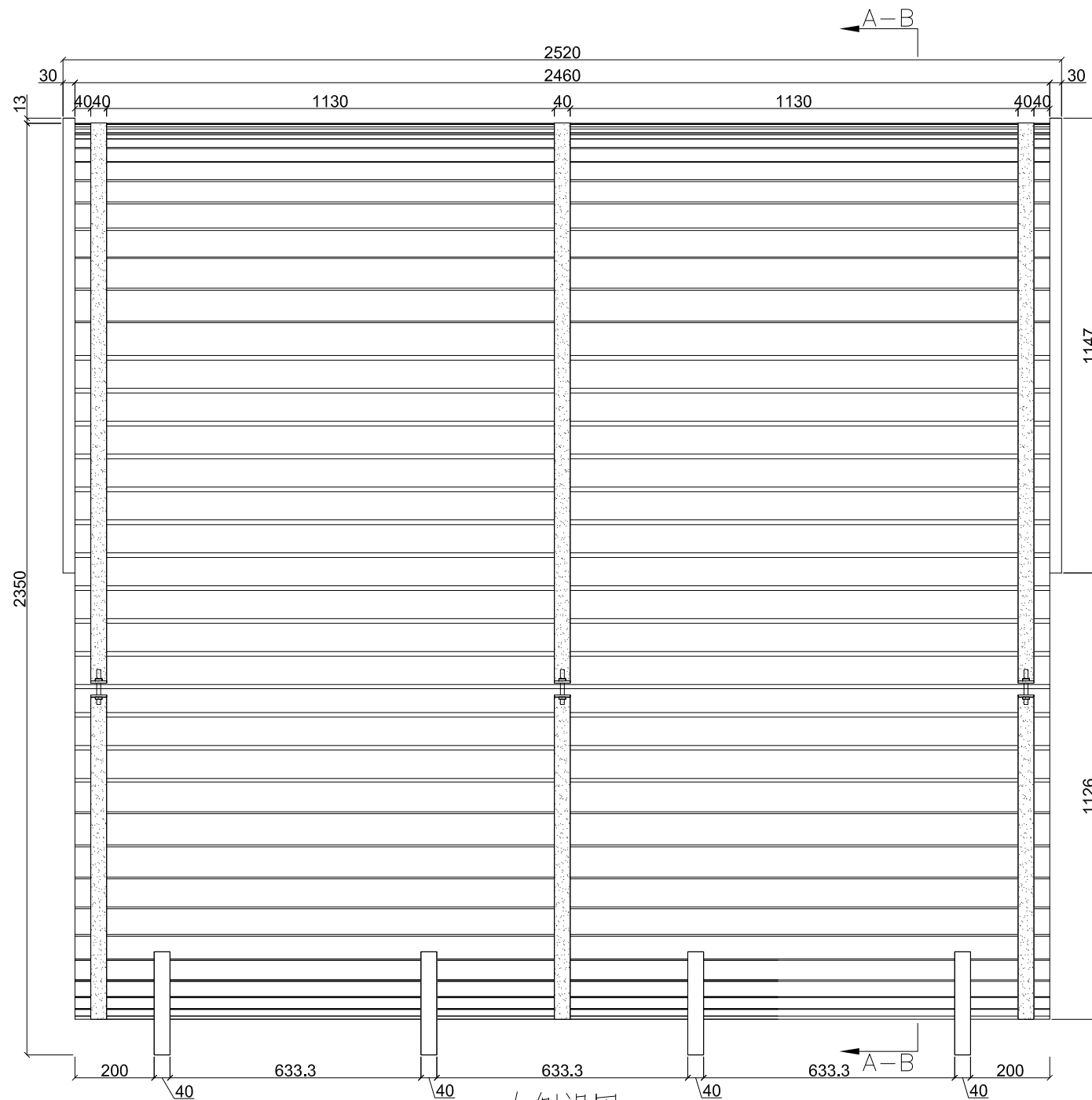
左侧视图
