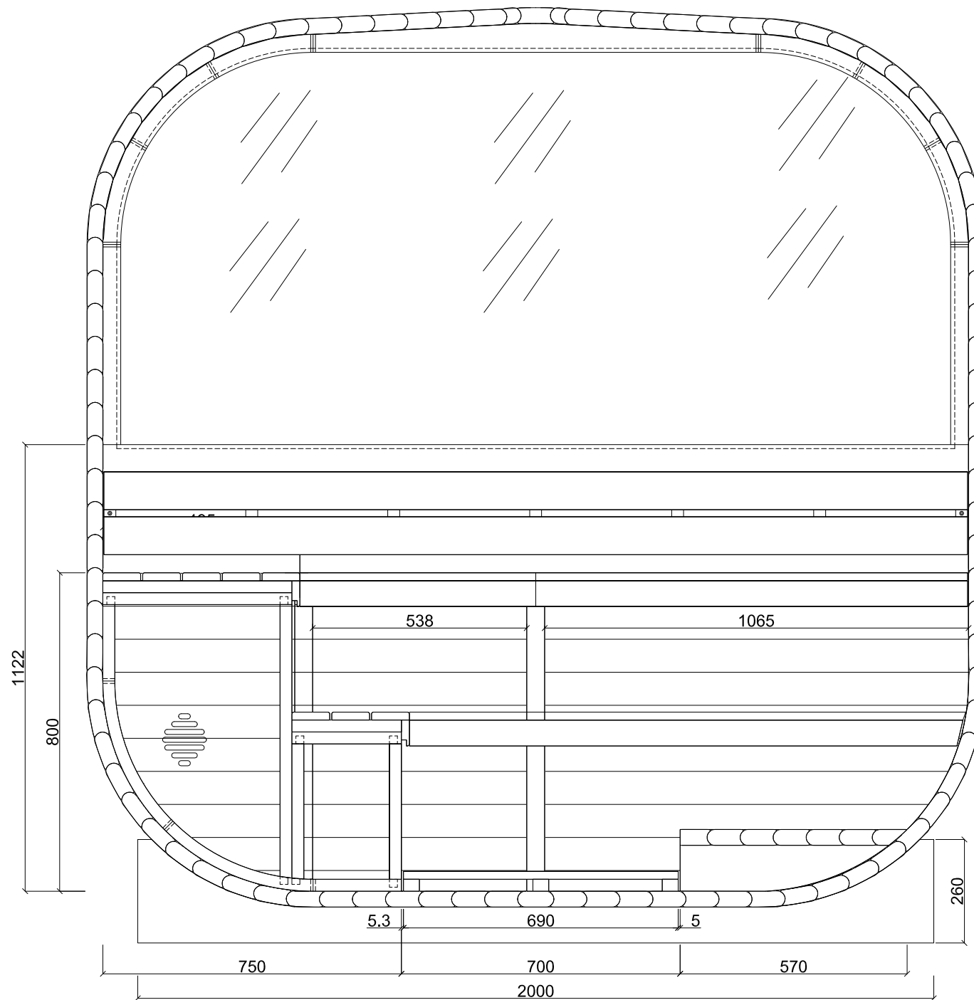
A-B剖视图
