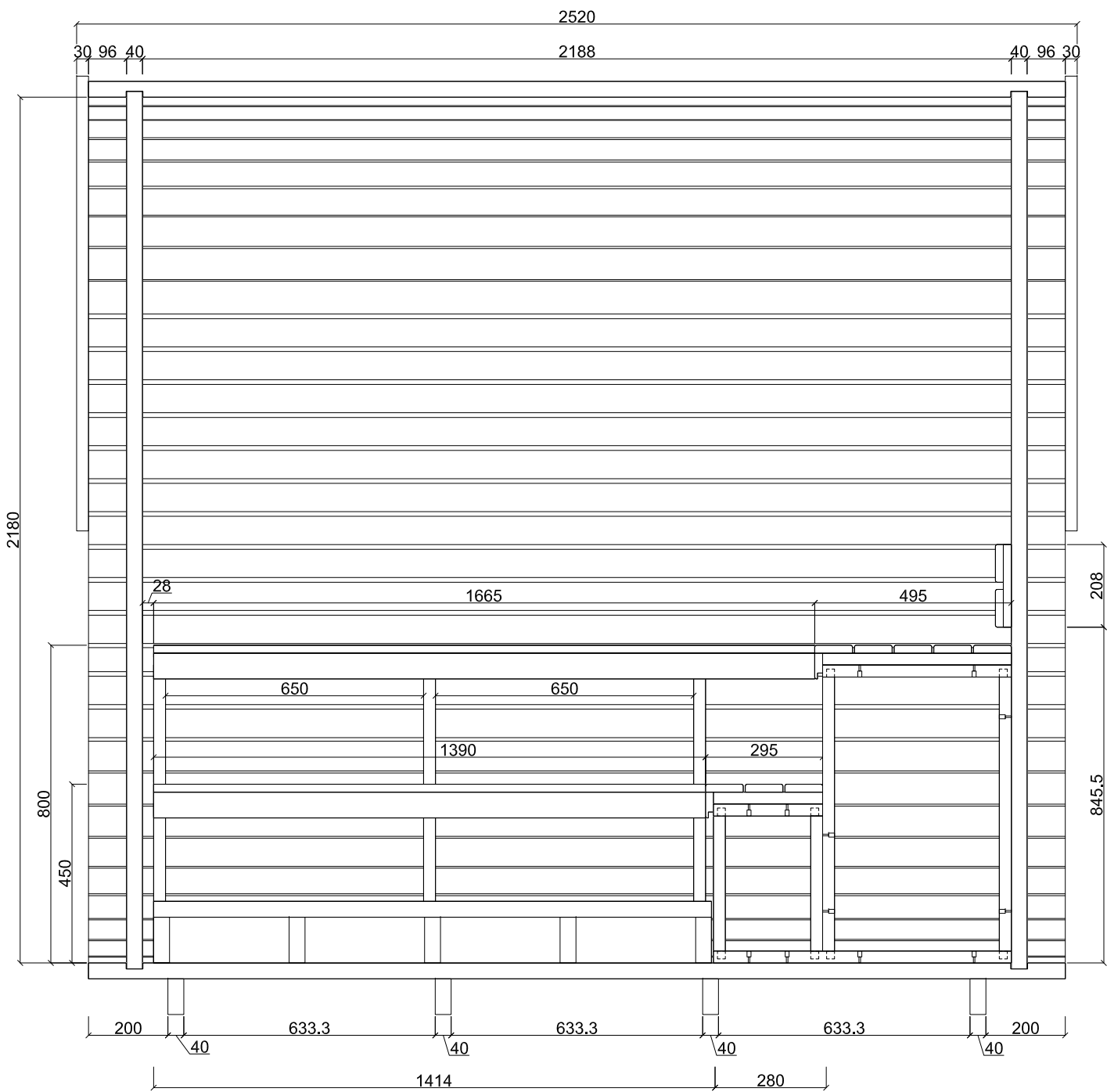
A-C 剖视图
