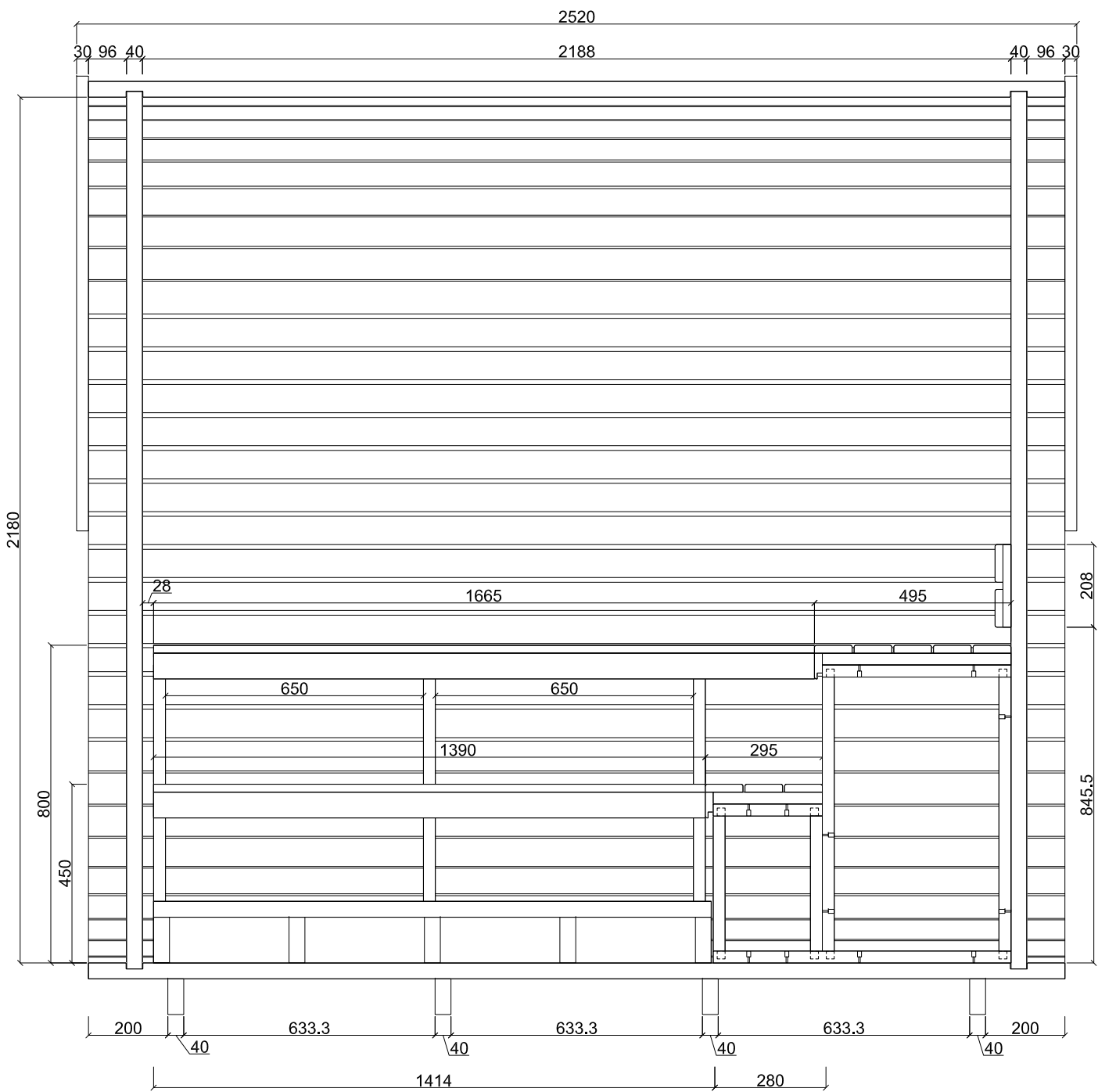
A-C 剖视图
