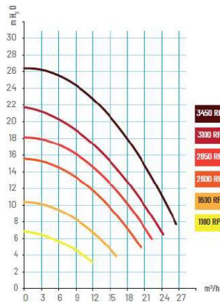
Sta-Rite VS2
